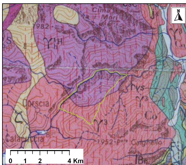
Figure 10 : Carte géologique de la Haute vallée de la Scala di Santa Regina (extrait de Rossi & Rouire 1980) jaune= périmètre de la ZPS ; bleu= granite hypersolvus à hastingsite-fayalite; orangé= granodiorite et monzogranite de Corse centrale
